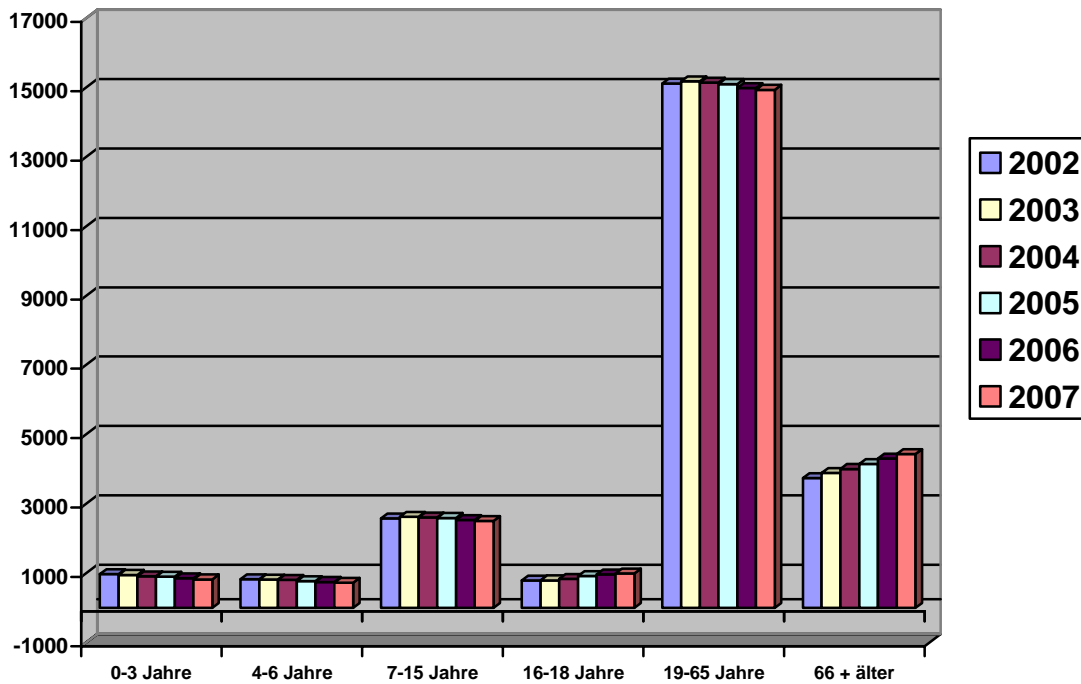
Altersstruktur
